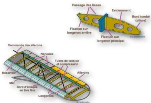
La structure de l'avion
